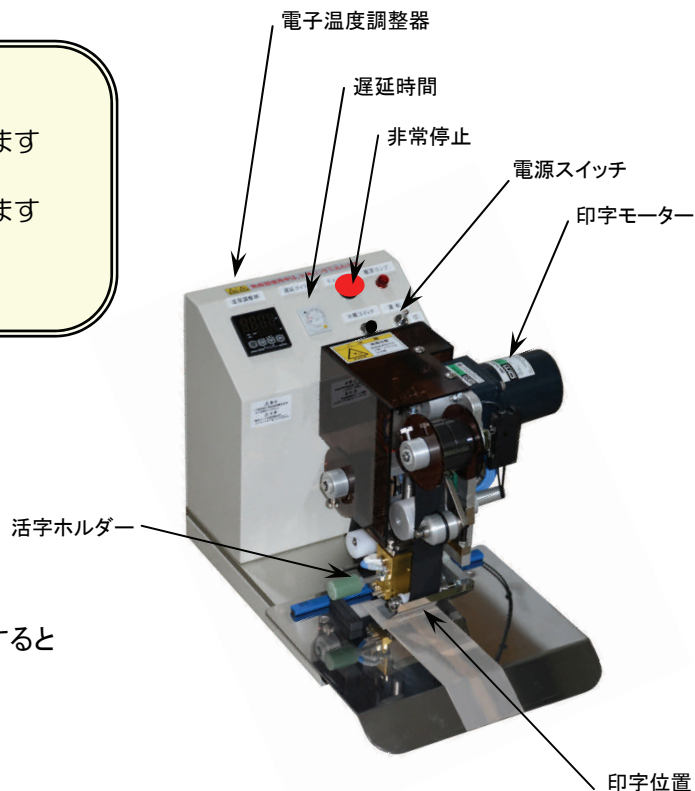
標準 2 列活字ホルダー
